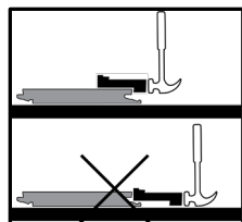
Position du bloc de tapement pour planchers de 12 mm
