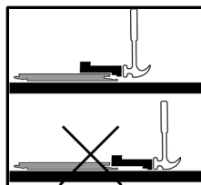
Position du bloc de tapement pour planchers de 8 mm
